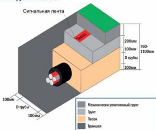
Многотрубная система
