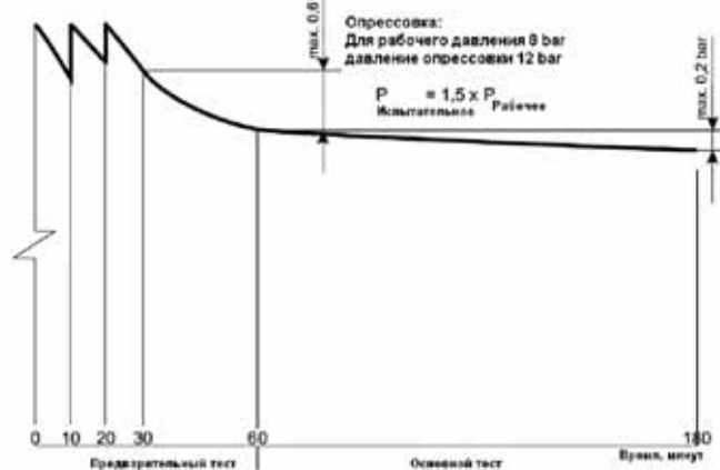
Диаграмма давления опрессовки (DIN 1988)
