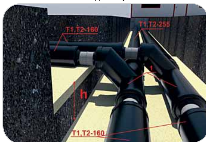
вид сбоку
